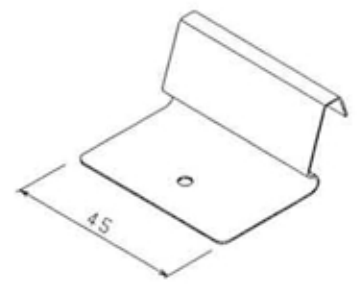
部分吊子( O. 8mm )
